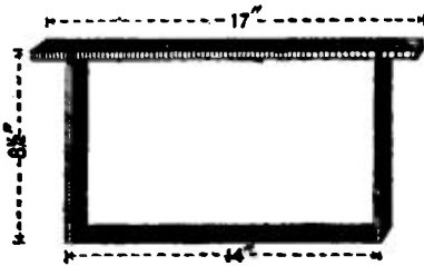
FIG. 14.—Standard Frame.
